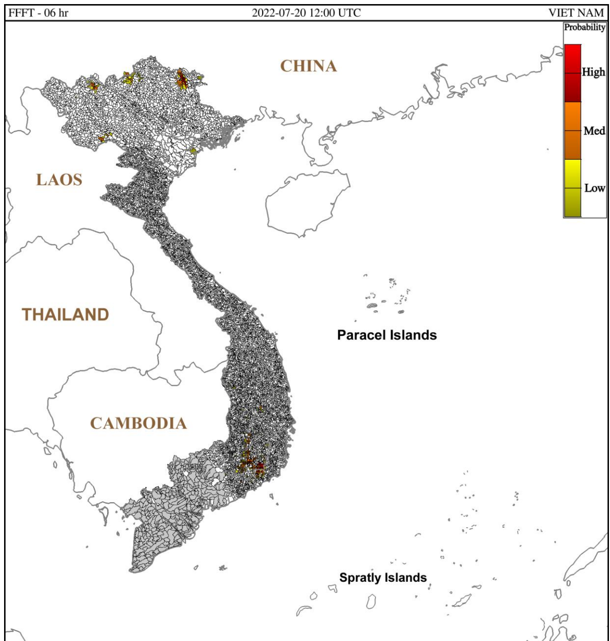
Hình 1. Nguy cơ lũ quét trong 6 giờ tới tại các lưu vực từ 19h ngày 20/07/2022 giờ địa phương
