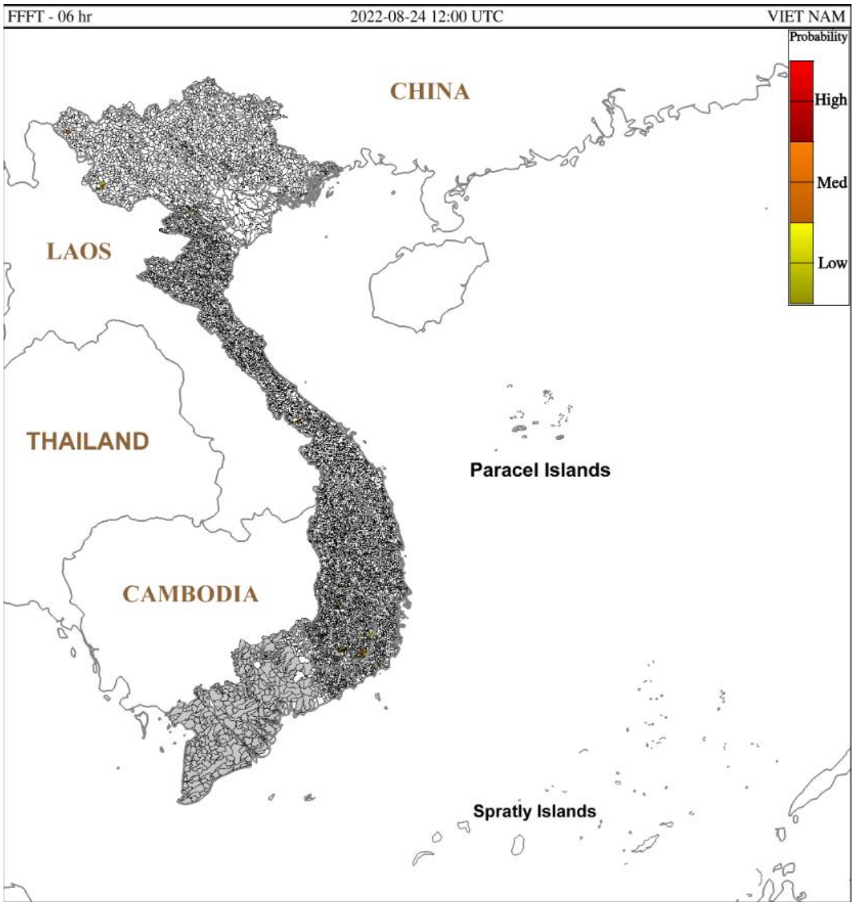
Hình 1. Nguy cơ lũ quét trong 6 giờ tới tại các lưu vực từ 19h ngày 24/08/2022 giờ địa phương
