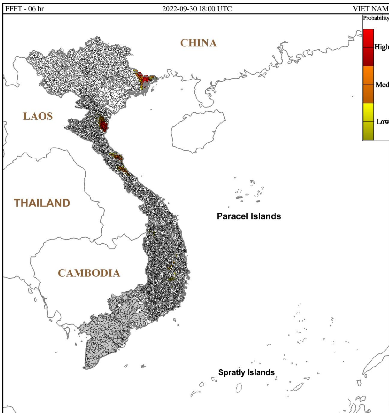
Hình 1. Nguy cơ lũ quét trong 6 giờ tới tại các lưu vực từ 01h ngày 01/10/2022 giờ địa phương
