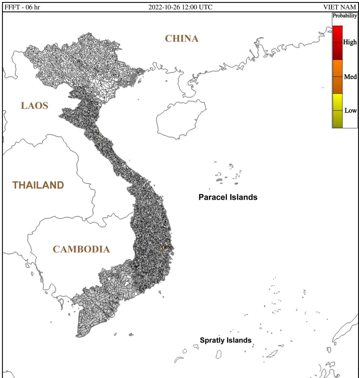
Hình 1. Nguy cơ lũ quét trong 6 giờ tới tại các lưu vực từ 19h ngày 26/10/2022 giờ địa phương
