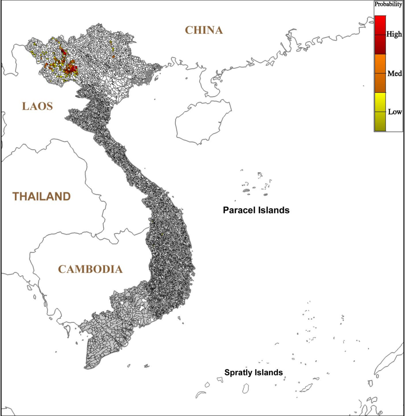
Hình 3: Nguy cơ lũ quét trong 6 giờ tới tại các lưu vực từ 07h ngày 12/08/2018 giờ địa phương
