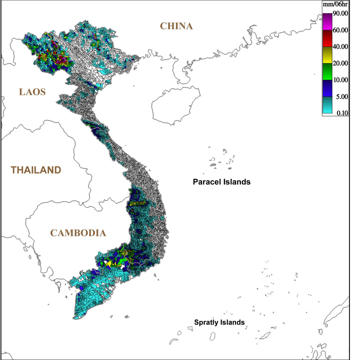
Hình 2: Dự báo lượng mưa trung bình lưu vực 6 giờ tính từ 07h ngày 12/08/2018 giờ địa phương
