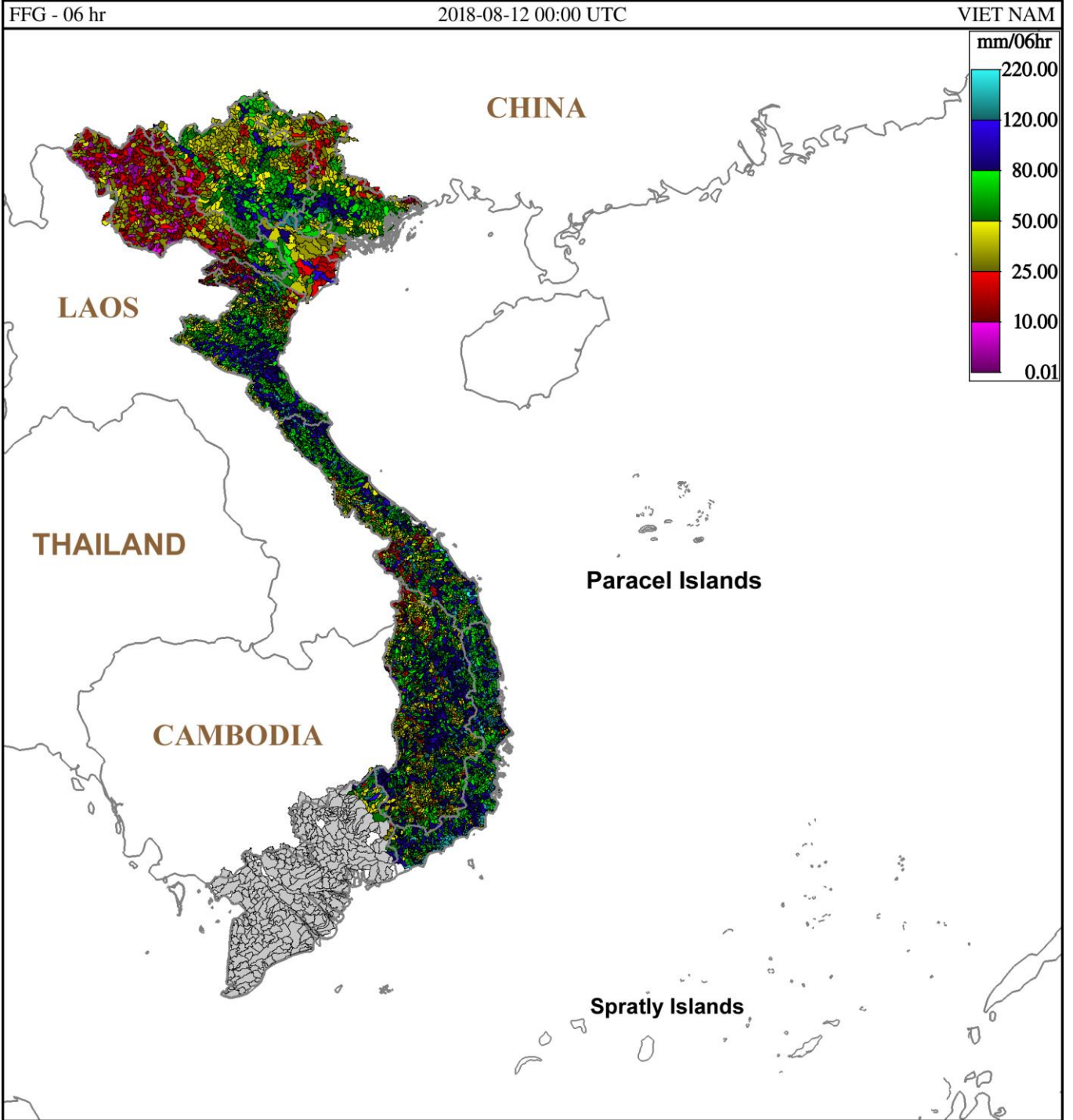
Hình 1. Ngưỡng mưa định hướng có khả năng sinh lũ quét trong 6 giờ tới tại các lưu vực từ 07h ngày 12/08/2018 giờ địa phương
