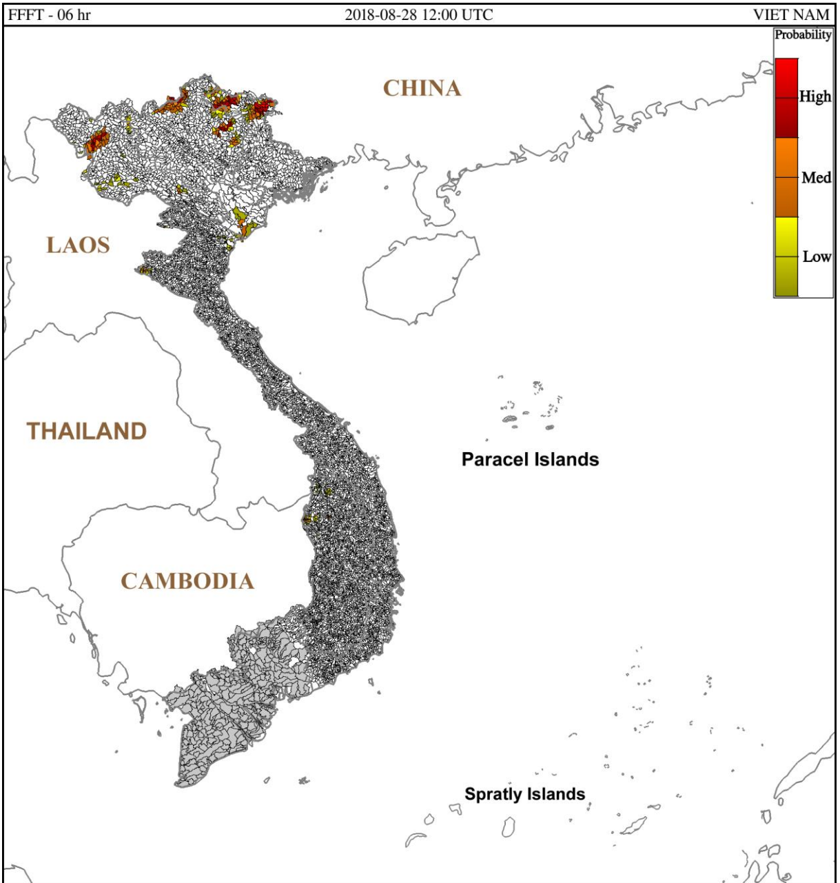
Hình 2: Nguy cơ lũ quét trong 6 giờ tới tại các lưu vực từ 19h ngày 28-08-2018 giờ địa phương
