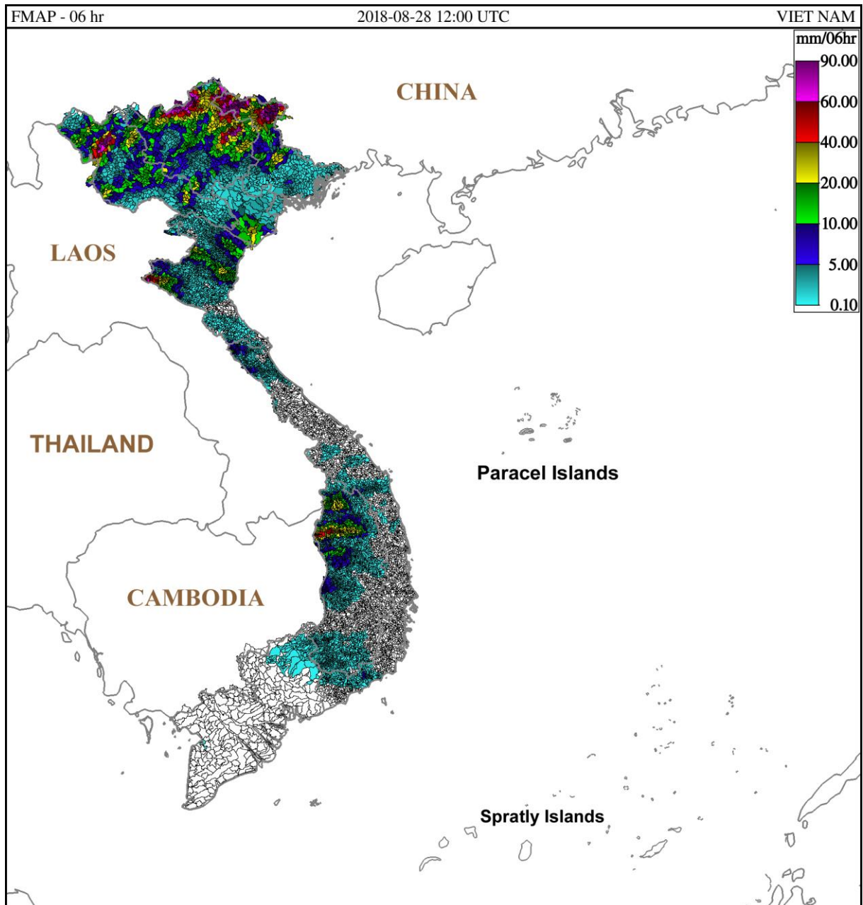
Hình 1: Dự báo lượng mưa trung bình lưu vực 6 giờ tính từ 19h ngày 28-08-2018 giờ địa phương
