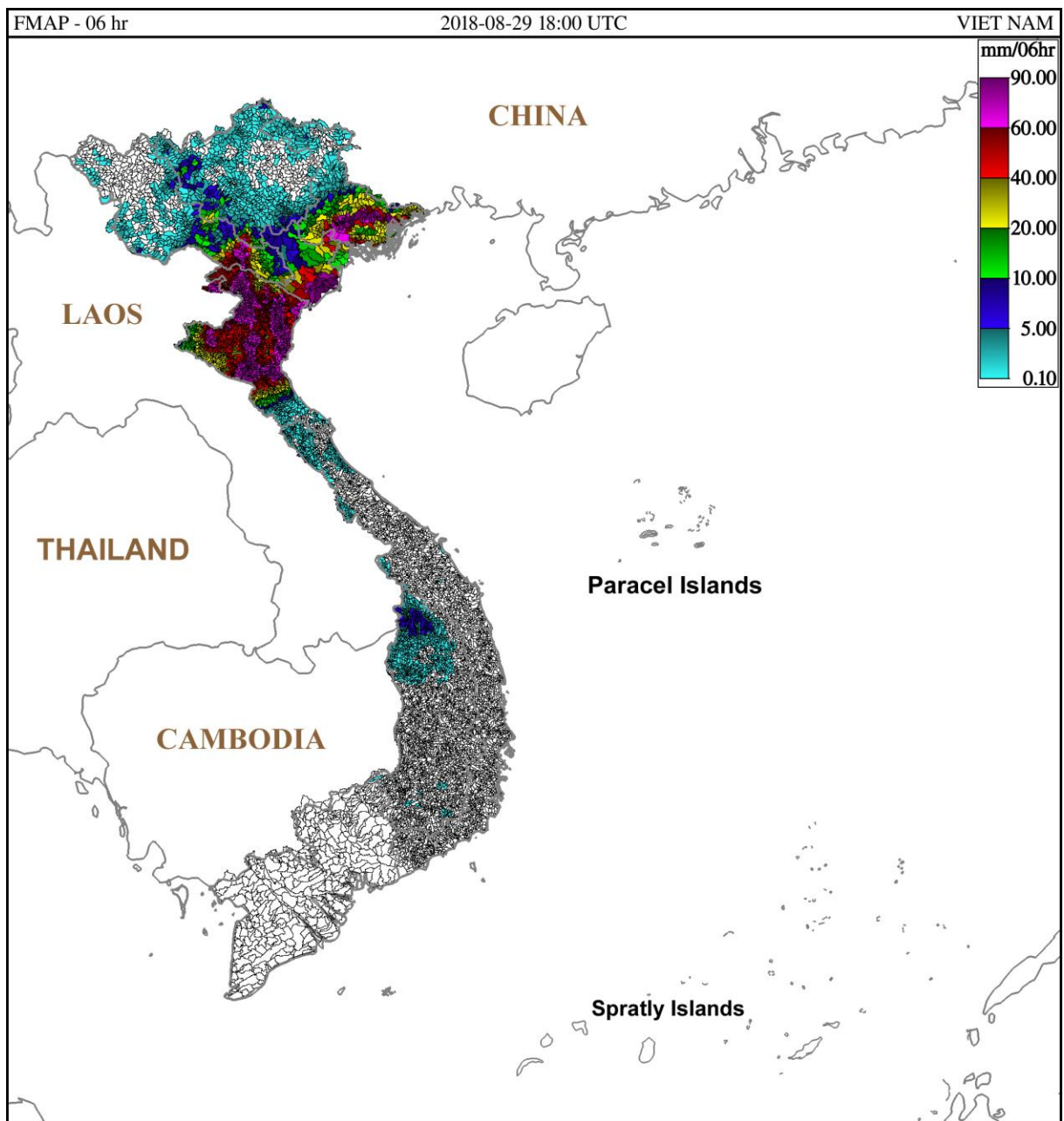
Hình 1: Dự báo lượng mưa trung bình lưu vực 6 giờ tính từ 01h ngày 30-8-2018 giờ địa phương
