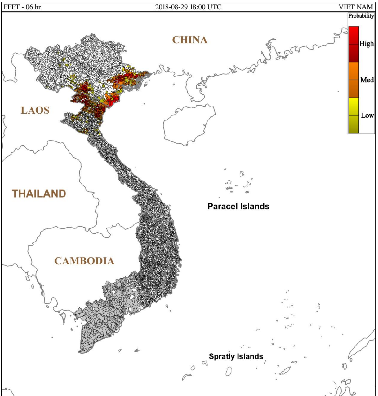
Hình 2: Nguy cơ lũ quét trong 6 giờ tới tại các lưu vực từ 01h ngày 30-8-2018 giờ địa phương
