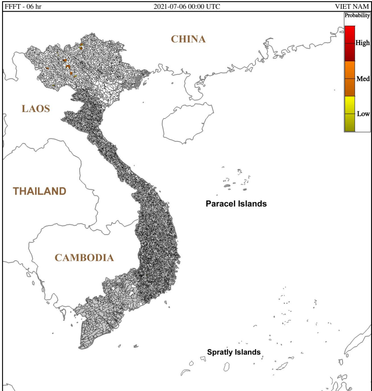
Hình 1. Nguy cơ lũ quét trong 6 giờ tới tại các lưu vực từ 07h ngày 06/7/2021 giờ địa phương
