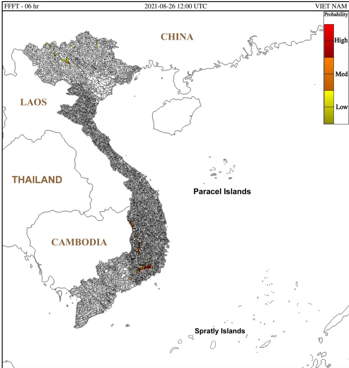
Hình 1. Nguy cơ lũ quét trong 6 giờ tới tại các lưu vực từ 19h ngày 26/8/2021 giờ địa phương
