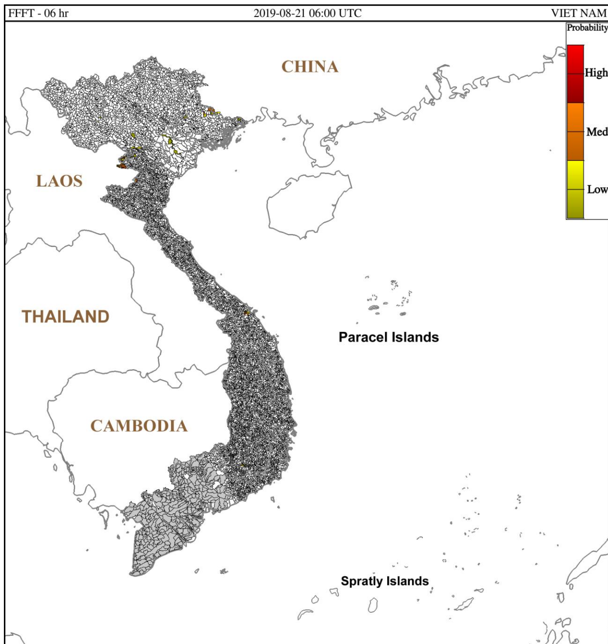
Hình 1: Nguy cơ lũ quét trong 6 giờ tới tại các lưu vực từ 13h ngày 21/08/2019 giờ địa phương
