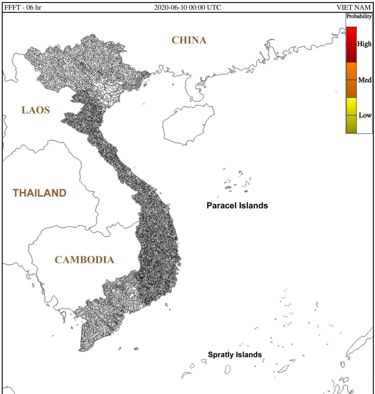
Hình 1: Nguy cơ lũ quét trong 6 giờ tới tại các lưu vực từ 07h ngày 10/06/2020 giờ địa phương
