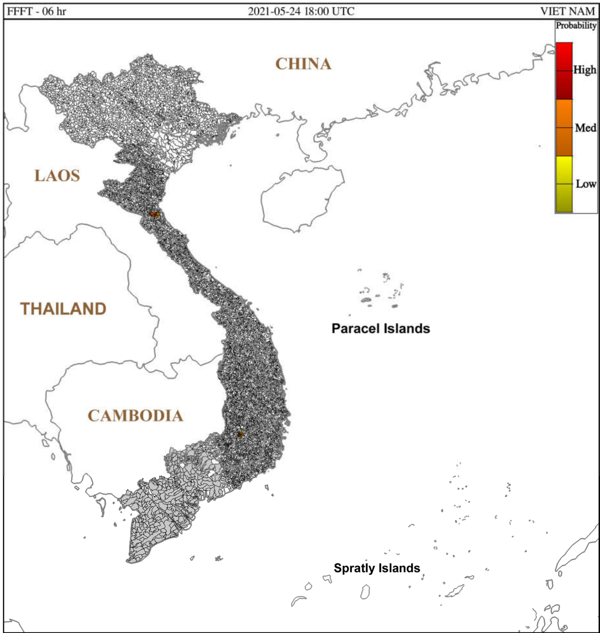
Hình 1. Nguy cơ lũ quét trong 6 giờ tới tại các lưu vực từ 01h ngày 25/05/2021 giờ địa phương
