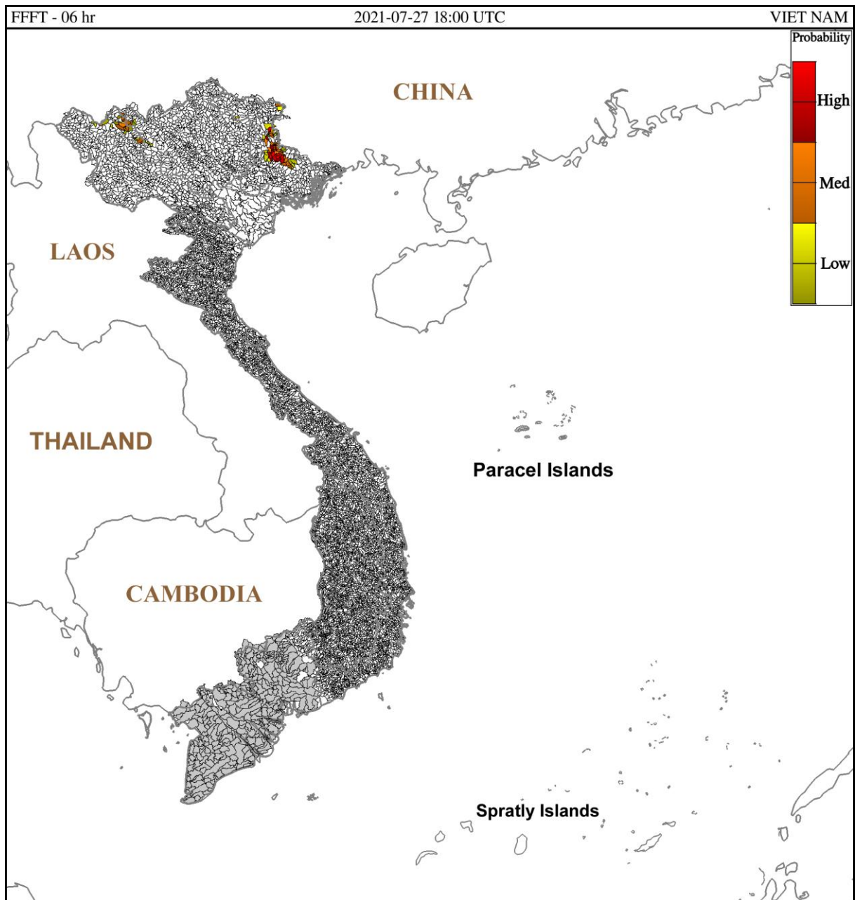
Hình 1. Nguy cơ lũ quét trong 6 giờ tới tại các lưu vực từ 01h ngày 28/07/2021 giờ địa phương
