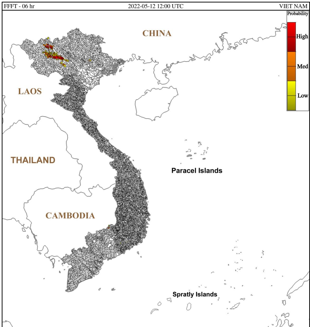
Hình 1. Nguy cơ lũ quét trong 6 giờ tới tại các lưu vực từ 19h ngày 12/05/2022 giờ địa phương
