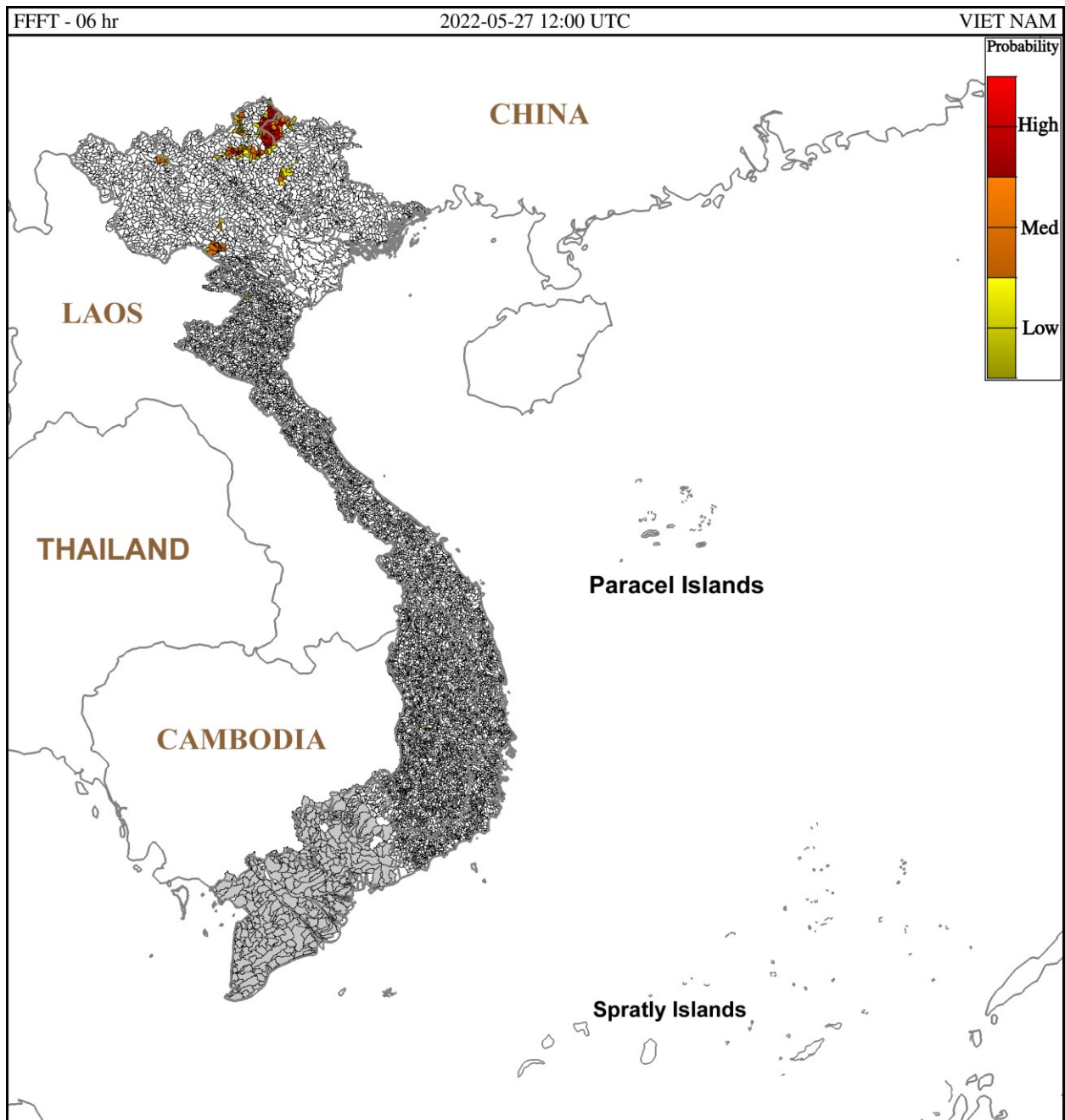
Hình 1. Nguy cơ lũ quét trong 6 giờ tới tại các lưu vực từ 19h ngày 27/5/2022 giờ địa phương
