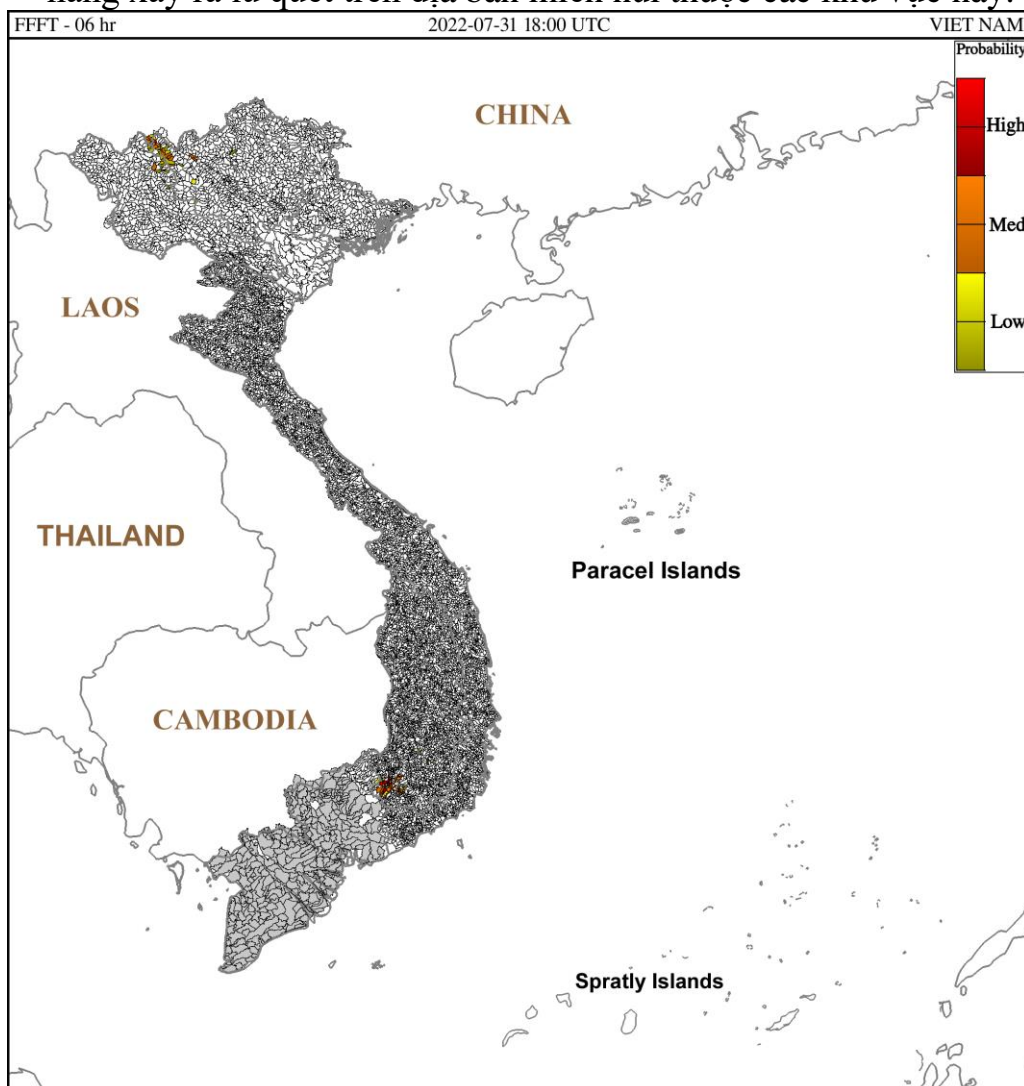
Hình 1. Nguy cơ lũ quét trong 6 giờ tới tại các lưu vực từ 01h ngày 01/08/2022 giờ địa phương
