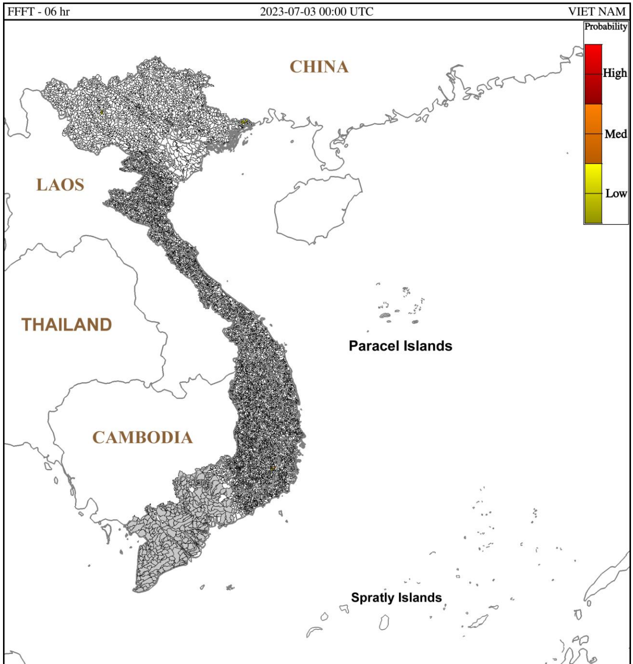
Hình 1. Nguy cơ lũ quét trong 6 giờ tới tại các lưu vực từ 7h ngày 03/07/2023 giờ địa phương
