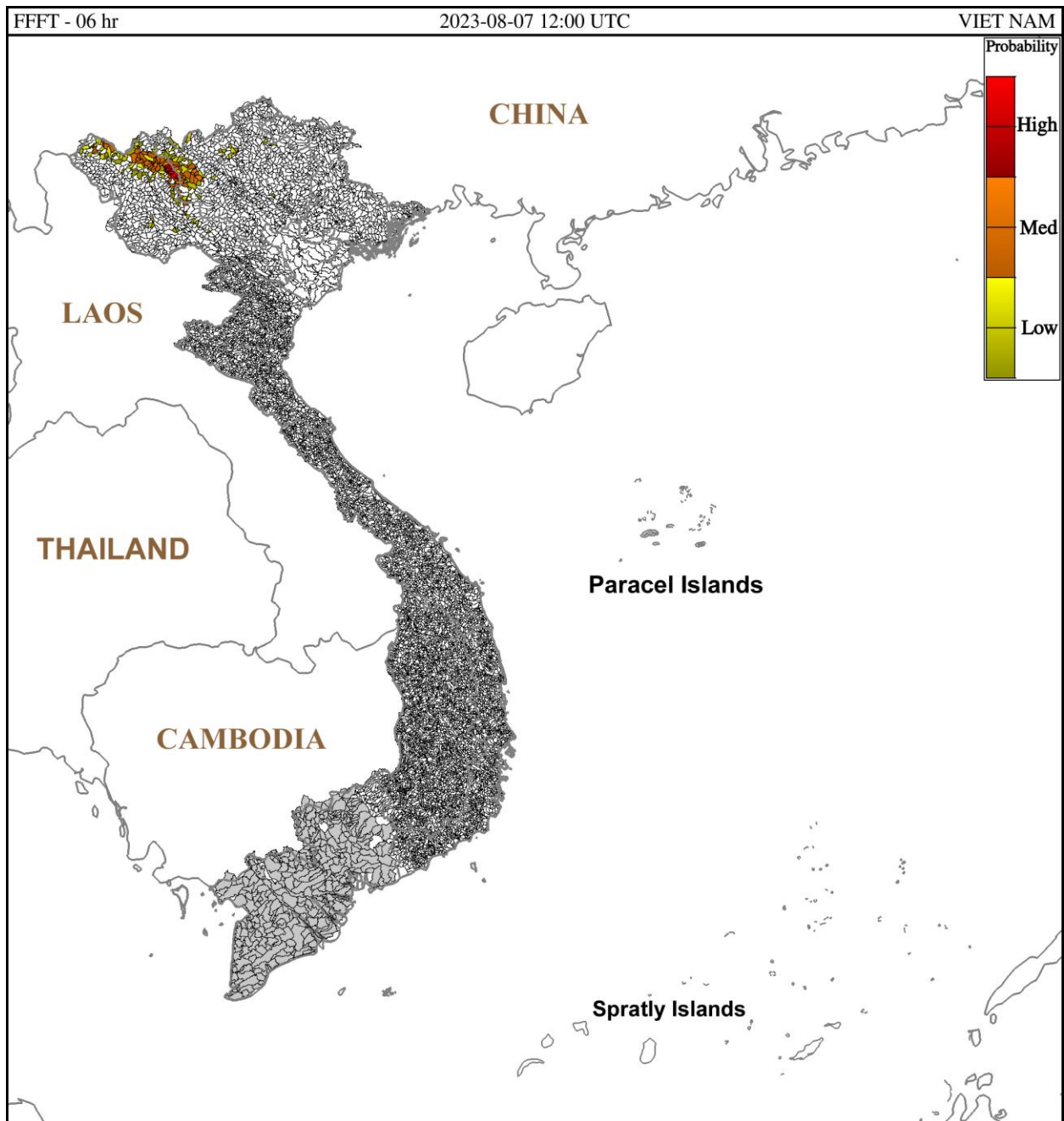
Hình 1. Nguy cơ lũ quét trong 6 giờ tới tại các lưu vực từ 19h ngày 07/8/2023 giờ địa phương
