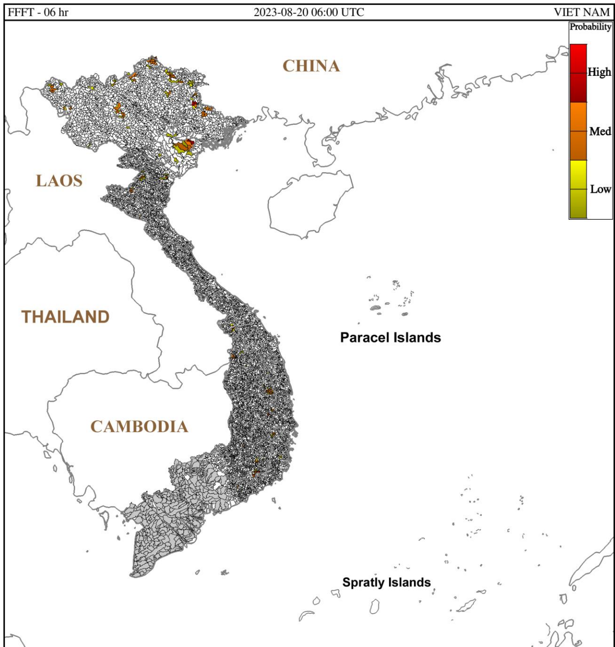
Hình 1. Nguy cơ lũ quét trong 6 giờ tới tại các lưu vực từ 13h ngày 20/08/2023 giờ địa phương
