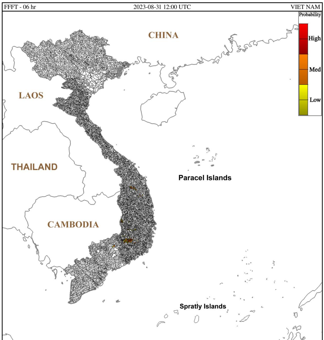
Hình 1. Nguy cơ lũ quét trong 6 giờ tới tại các lưu vực từ 19 ngày 31/8/2023 giờ địa phương
