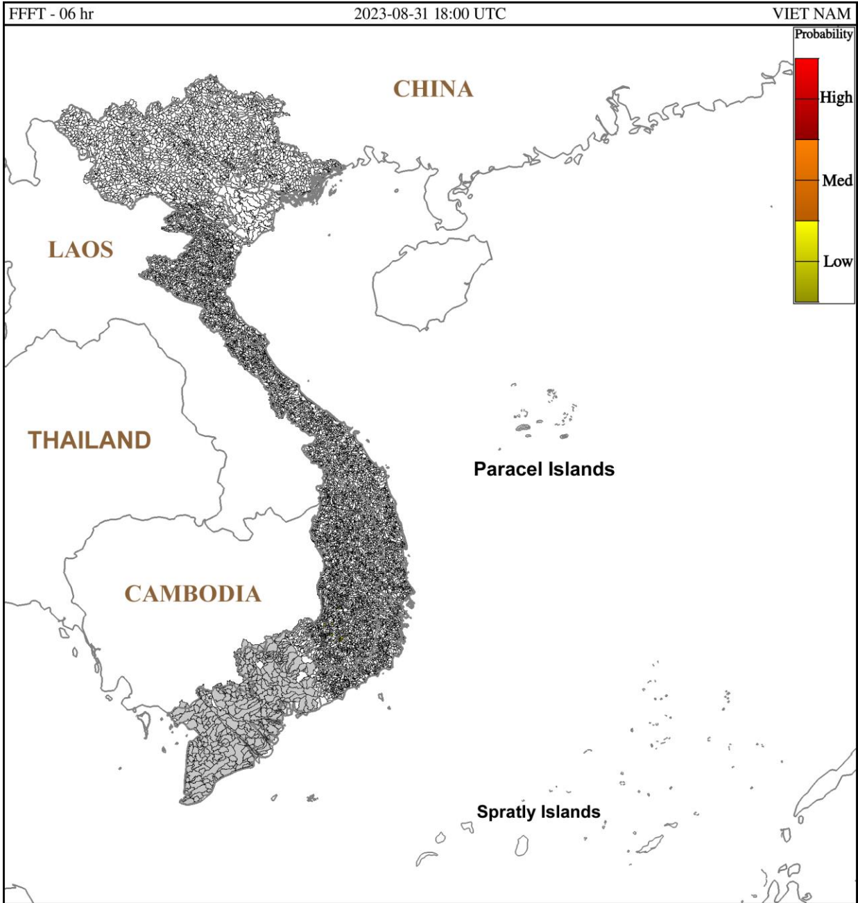
Hình 1. Nguy cơ lũ quét trong 6 giờ tới tại các lưu vực từ 01h ngày 01/9/2023 giờ địa phương
