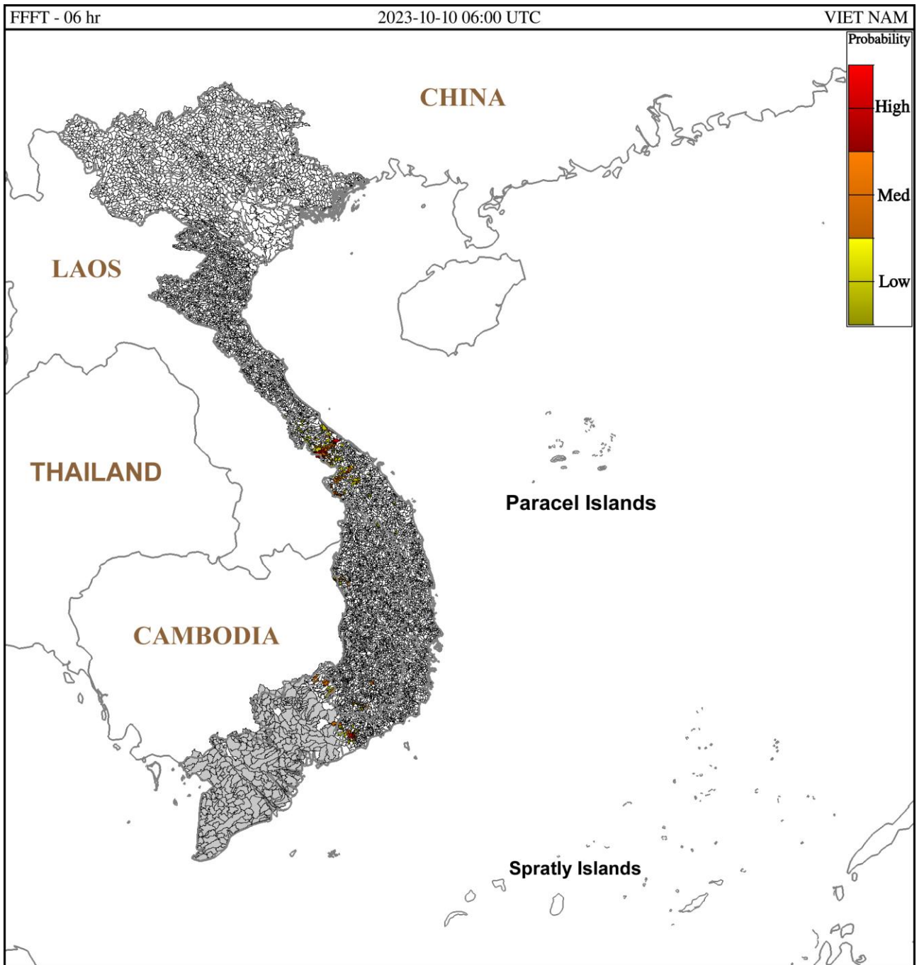
Hình 1. Nguy cơ lũ quét trong 6 giờ tới tại các lưu vực từ 13h ngày 10/10/2023 giờ địa phương
