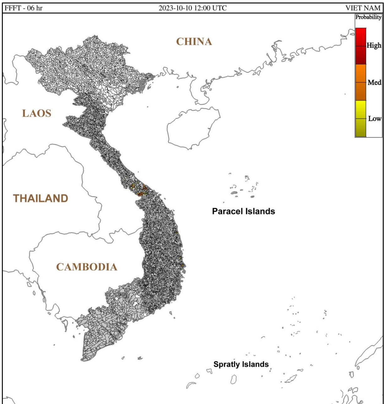
Hình 1. Nguy cơ lũ quét trong 6 giờ tới tại các lưu vực từ 19h ngày 10/10/2023 giờ địa phương
