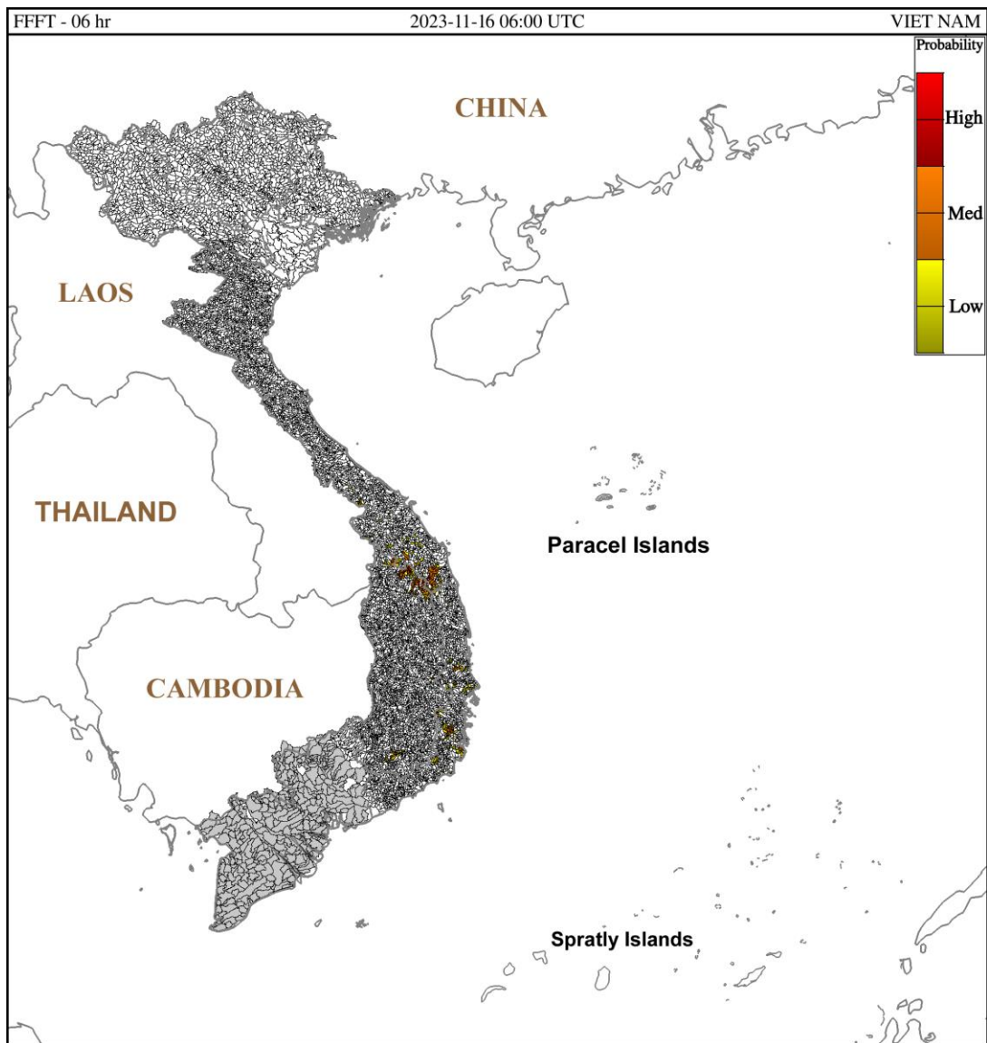
Hình 1. Nguy cơ lũ quét trong 6 giờ tới tại các lưu vực từ 13h ngày 16/11/2023 giờ địa phương
