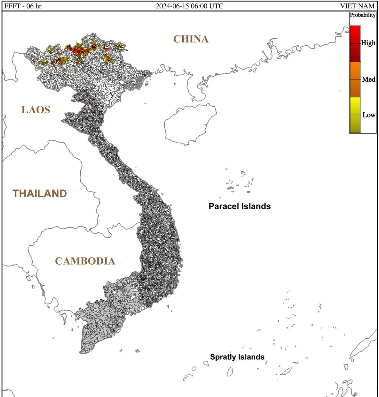
Hình 1. Nguy cơ lũ quét trong 6 giờ tới tại các lưu vực từ 13h ngày 15/6/2024 giờ địa phương
