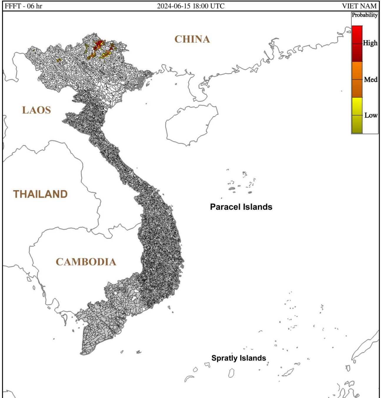
Hình 1. Nguy cơ lũ quét trong 6 giờ tới tại các lưu vực từ 01h ngày 16/6/2024 giờ địa phương
