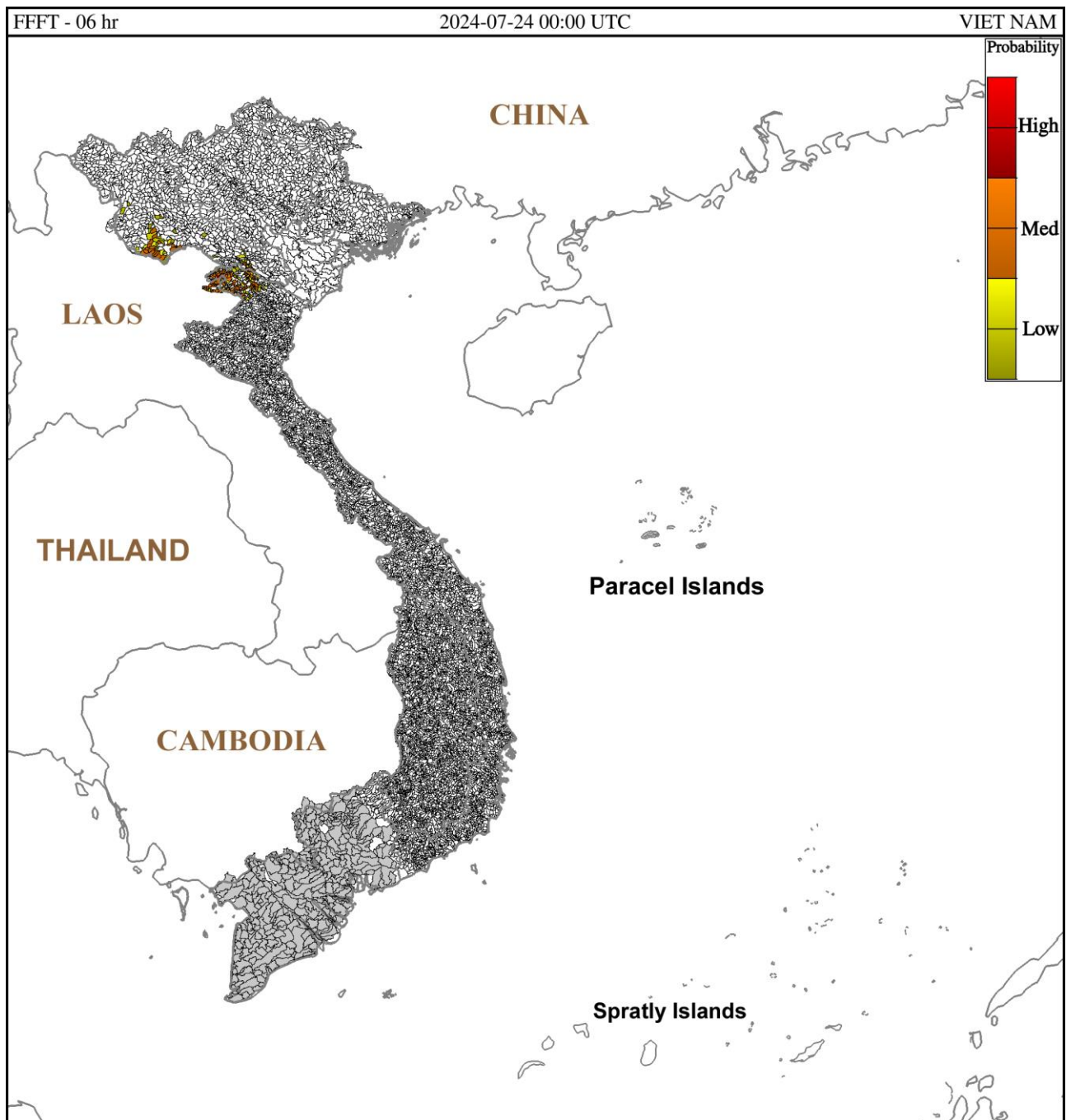
Hình 1: Nguy cơ lũ quét trong 6 giờ tới tại các lưu vực từ 07h ngày 24/07/2024 giờ địa phương
