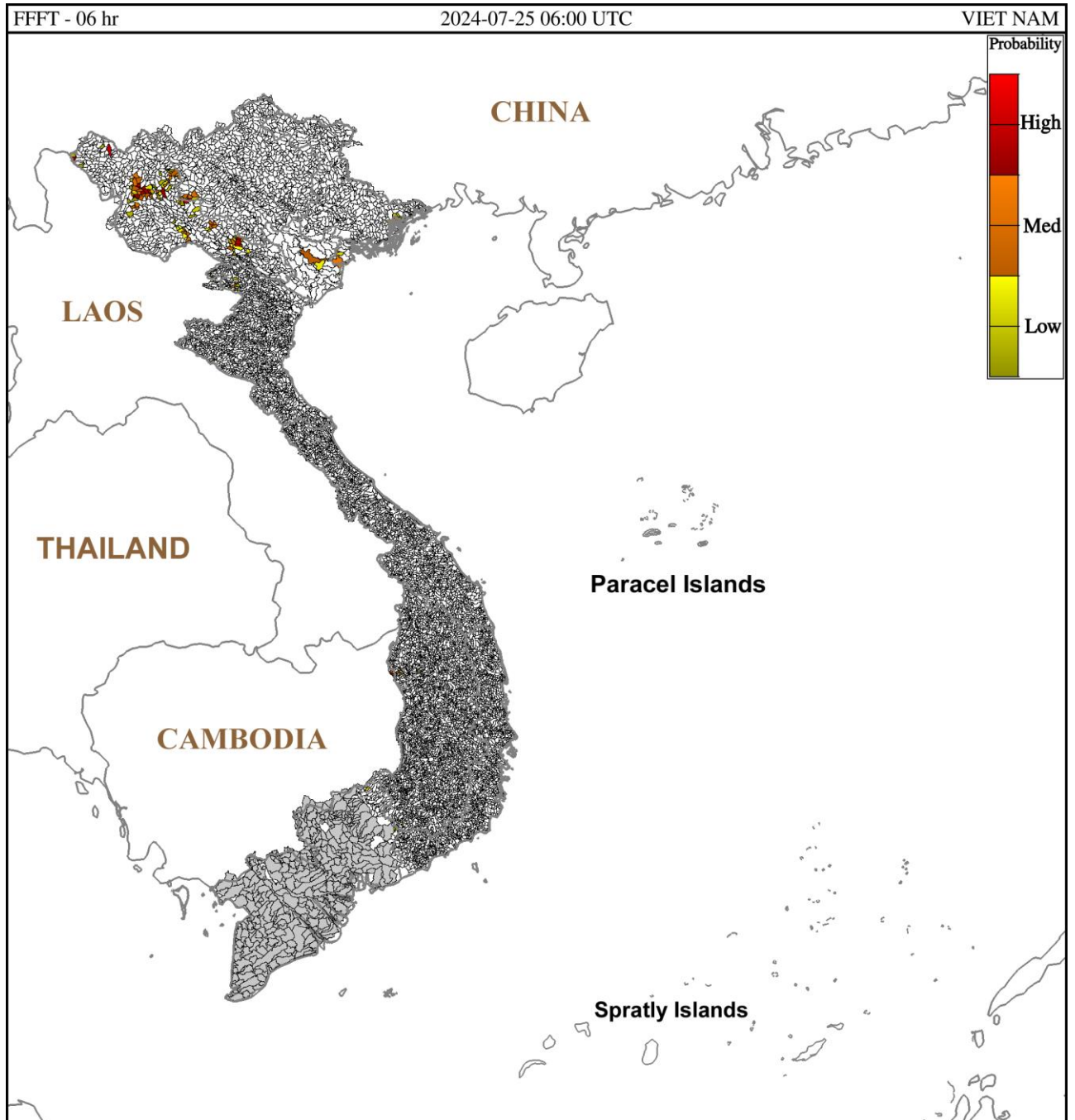
Hình 1: Nguy cơ lũ quét trong 6 giờ tới tại các lưu vực từ 13h ngày 25/07/2024 giờ địa phương
