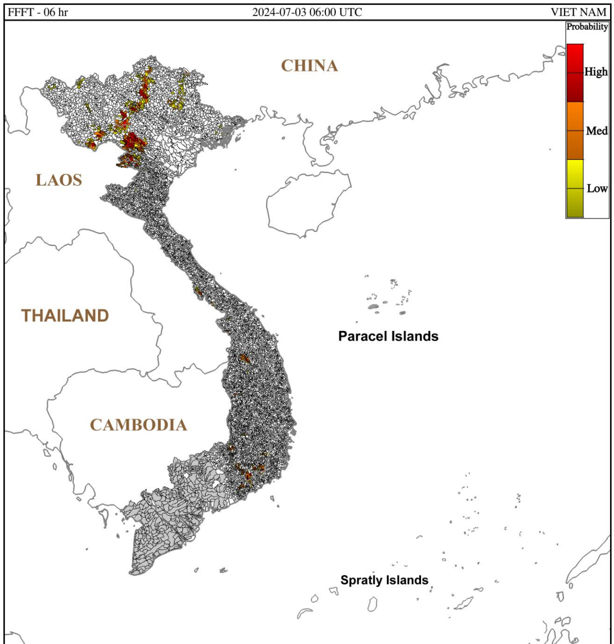
Hình 1. Nguy cơ lũ quét trong 6 giờ tới tại các lưu vực từ 13h ngày 03/7/2024 giờ địa phương
