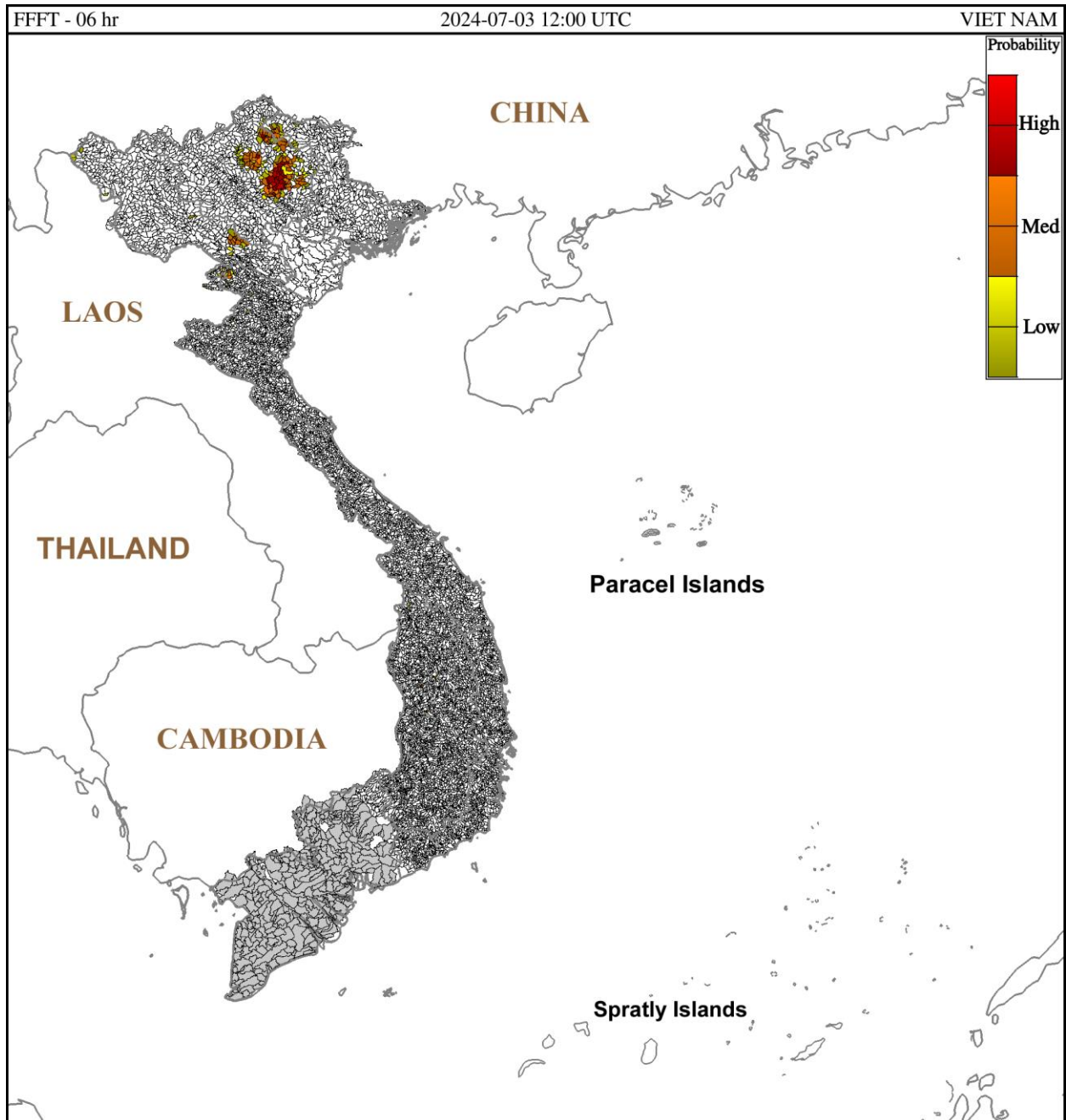
Hình 1. Nguy cơ lũ quét trong 6 giờ tới tại các lưu vực từ 19h ngày 03/7/2024 giờ địa phương
