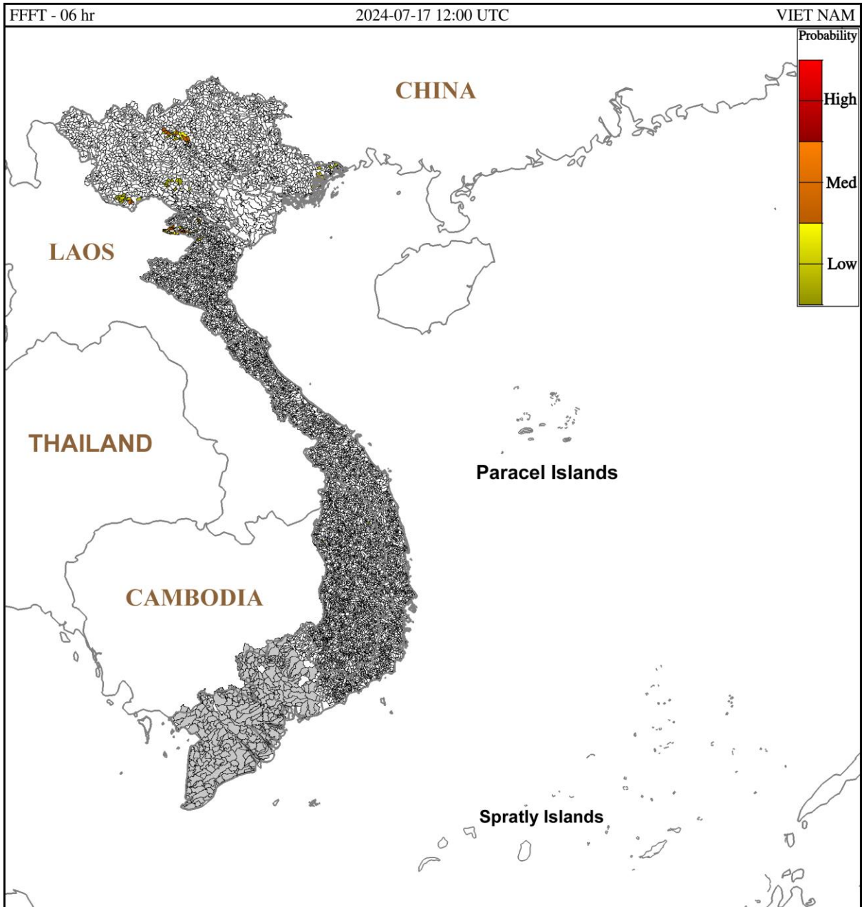
Hình 1. Nguy cơ lũ quét trong 6 giờ tới tại các lưu vực từ 19h ngày 17/7/2024 giờ địa phương
