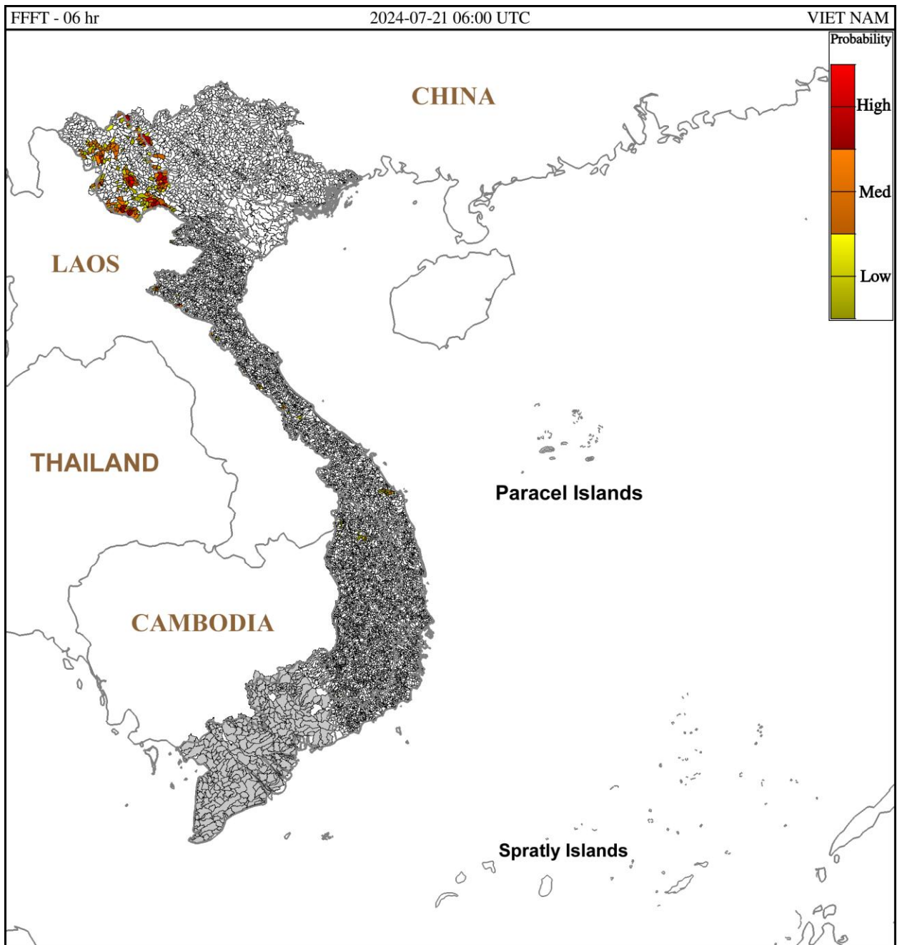
Hình 1. Nguy cơ lũ quét trong 6 giờ tới tại các lưu vực từ 13h ngày 21/7/2024 giờ địa phương
