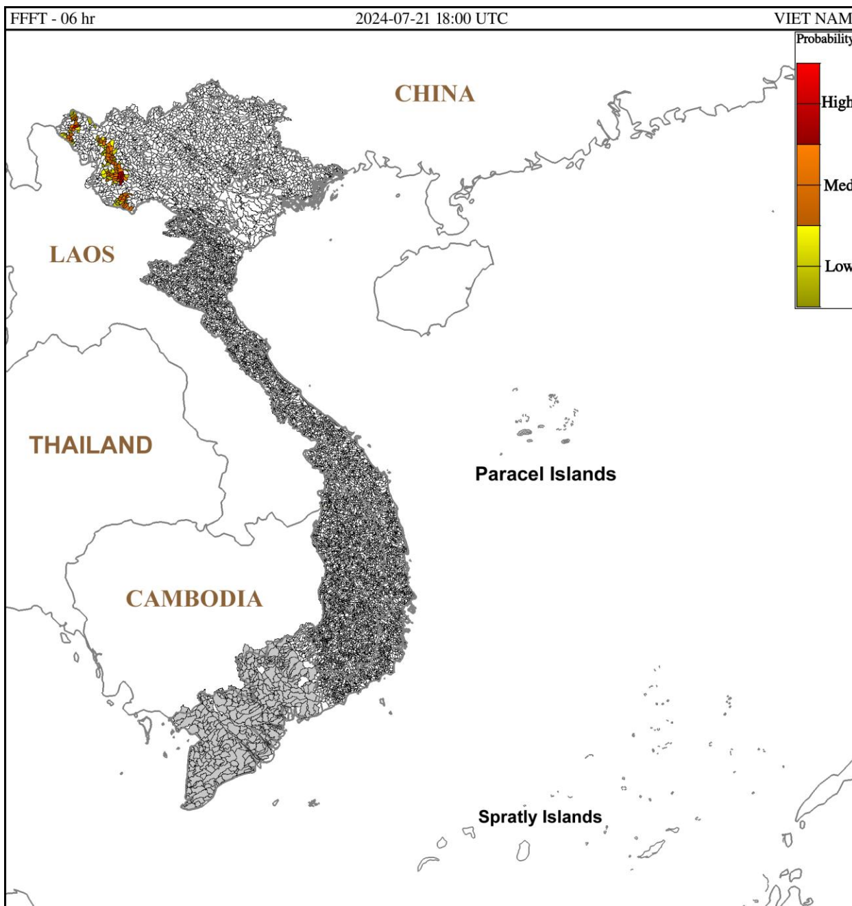
Hình 1. Nguy cơ lũ quét trong 6 giờ tới tại các lưu vực từ 01h ngày 22/7/2024 giờ địa phương
