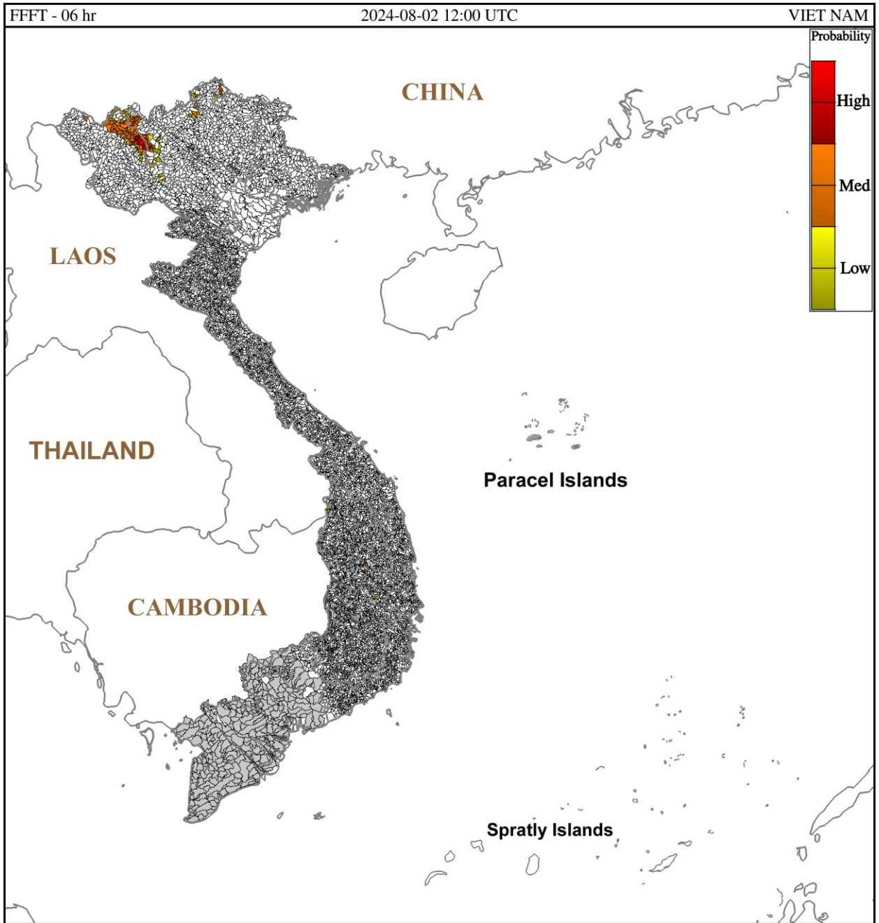
Hình 1: Nguy cơ lũ quét trong 6 giờ tới tại các lưu vực từ 19h ngày 02/08/2024 giờ địa phương
