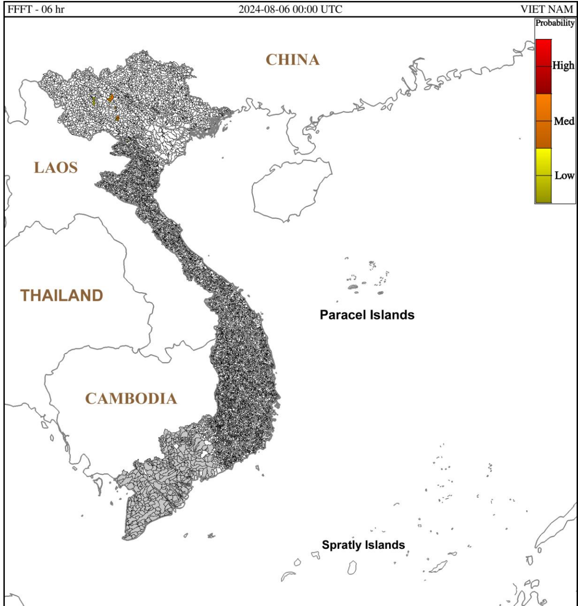
Hình 1. Nguy cơ lũ quét trong 6 giờ tới tại các lưu vực từ 07h ngày 06/8/2024 giờ địa phương
