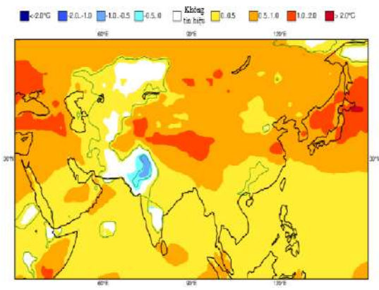
Hình 2.4. Dự báo chuẩn sai nhiệt độ mùa 3 tháng 8-10 năm 2025 (Nguồn: http://www.ecmwf.int )
