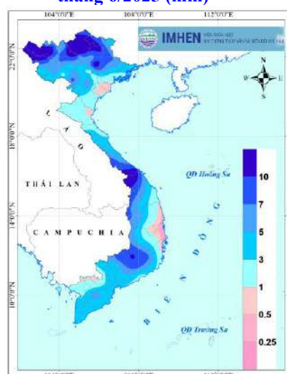
Hình 1.23. Phân bố chỉ số ẩm tháng 6/2025
