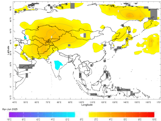
Hình 1.4. Phân bố chuẩn sai NĐTB mùa 3 tháng 4-6 năm 2025 ( ^{\circ}\text{C} ) trên khu vực châu Á (Nguồn: http://iridl.ldeo.columbia.edu/ )
