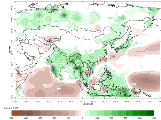
Hình 1.5. Phân bố chuẩn sai TLM mùa 3 tháng 4-6 năm 2025 (mm) trên khu vực châu Á (Nguồn: http://iridl.ldeo.columbia.edu/ )
