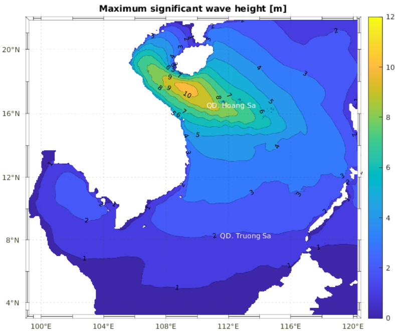
Phân bố chiều cao sóng có nghĩa lớn nhất với hạn dự báo 72 giờ
