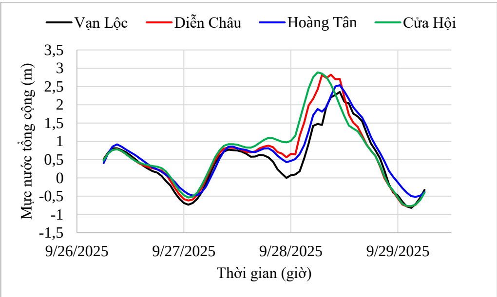
Biến trình mức nước tổng cộng trong 72 giờ
