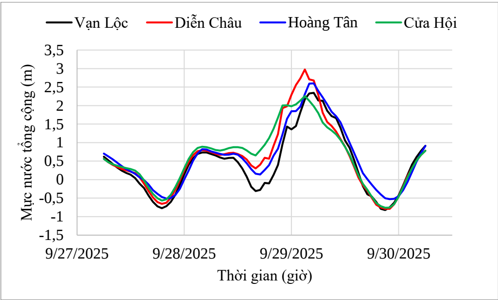
Biến trình mực nước tổng cộng trong 72 giờ
