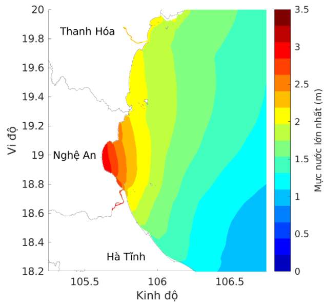
Phân bố mực nước tổng cộng lớn nhất với hạn dự báo 72h
