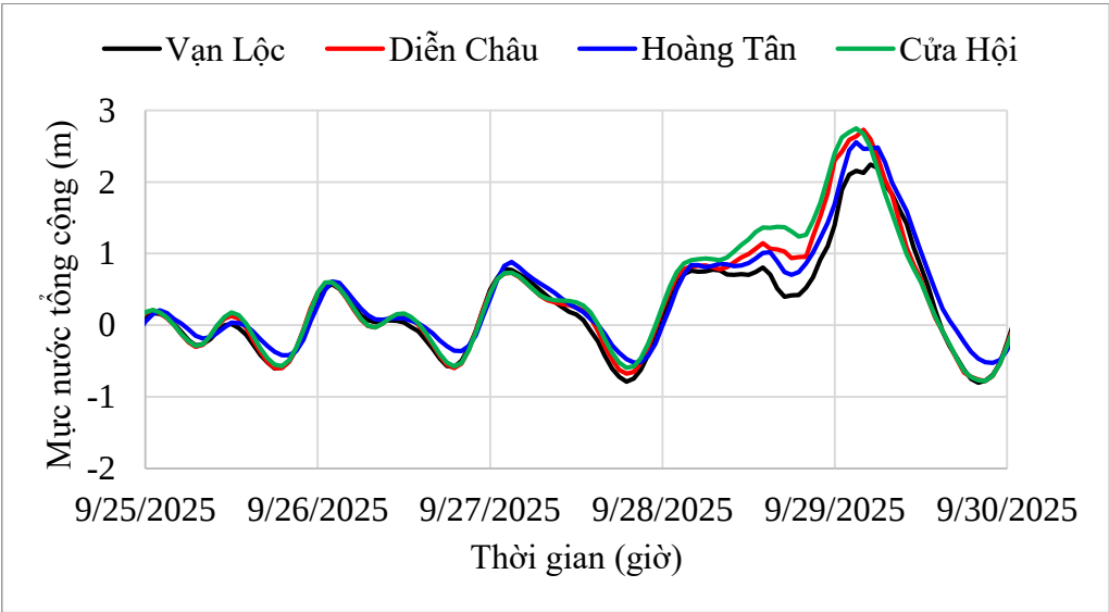
Biến trình mức nước tổng cộng từ ngày 25-30/9/2025
