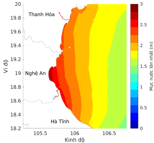
Phân bố mực nước tổng cộng lớn nhất với hạn dự báo 72h
