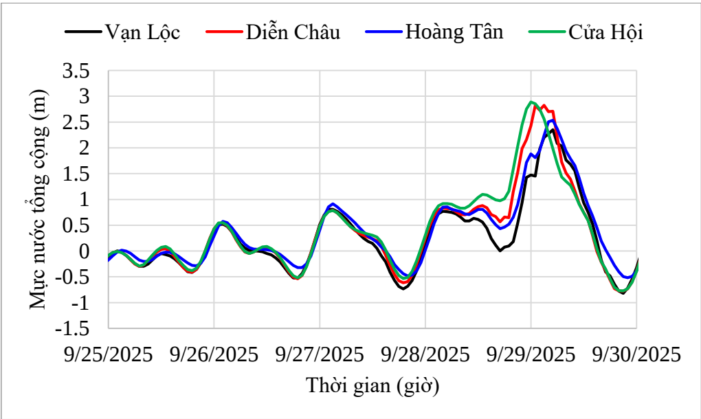
Biến trình mực nước tổng cộng từ ngày 25-30/9/2025
