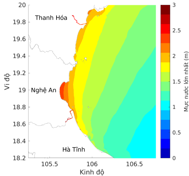
Phân bố mức nước tổng cộng lớn nhất với hạn dự báo 72h
