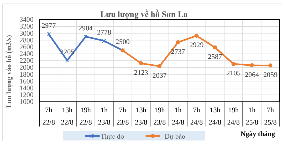
Hình 5: Lưu lượng hồ Sơn La
