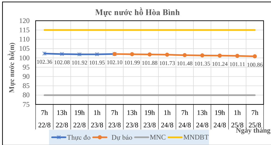
Hình 8: Mức nước hồ Hòa Bình
