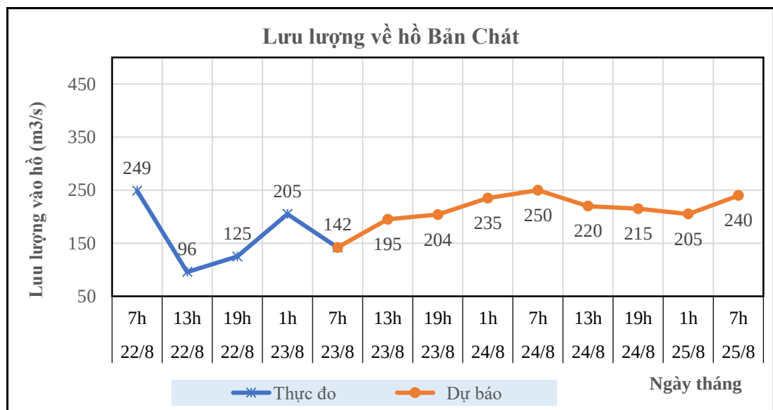
Hình 13: Lưu lượng hồ Bản Chát
