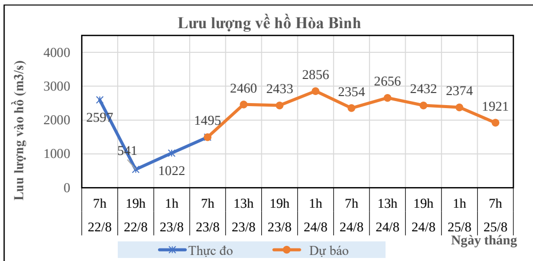
Hình 7: Lưu lượng hồ Hòa Bình
