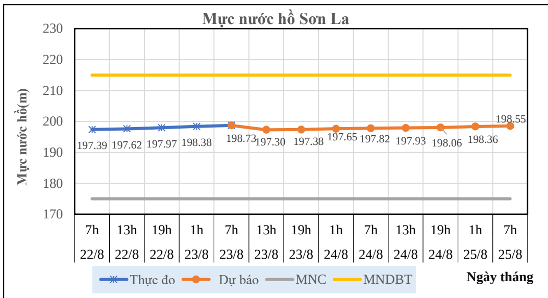
Hình 6: Mức nước hồ Sơn La
