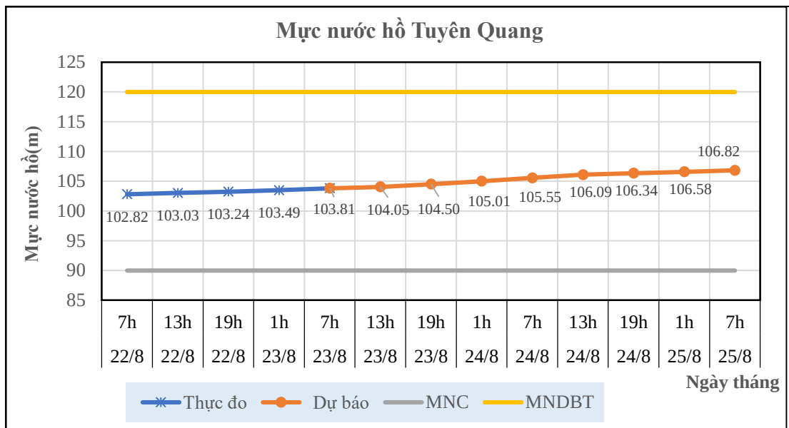
Hình 10: Mức nước hồ Tuyên Quang
