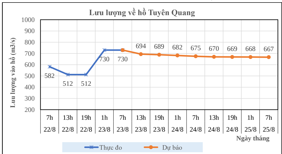
Hình 9: Lưu lượng hồ Tuyên Quang
