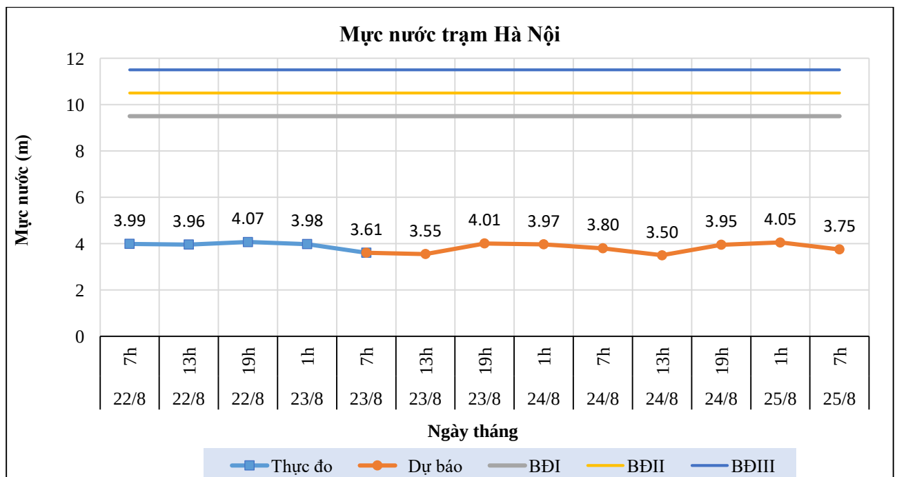
Hình 3: Mức nước trạm Hà Nội
